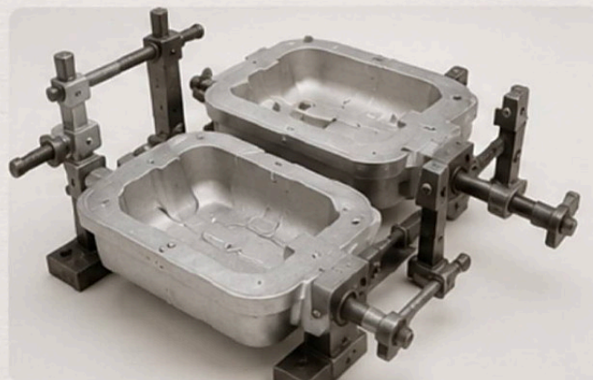
MOULAGE EN COQUILLE Coquille chauffée et assemblée.
