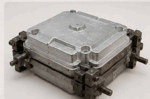
MOULAGE EN COQUILLE Coquille prête pour la coulée.
