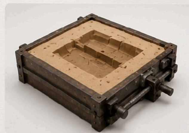
MOULAGE AU SABLE Moule prêt pour la coulée.
